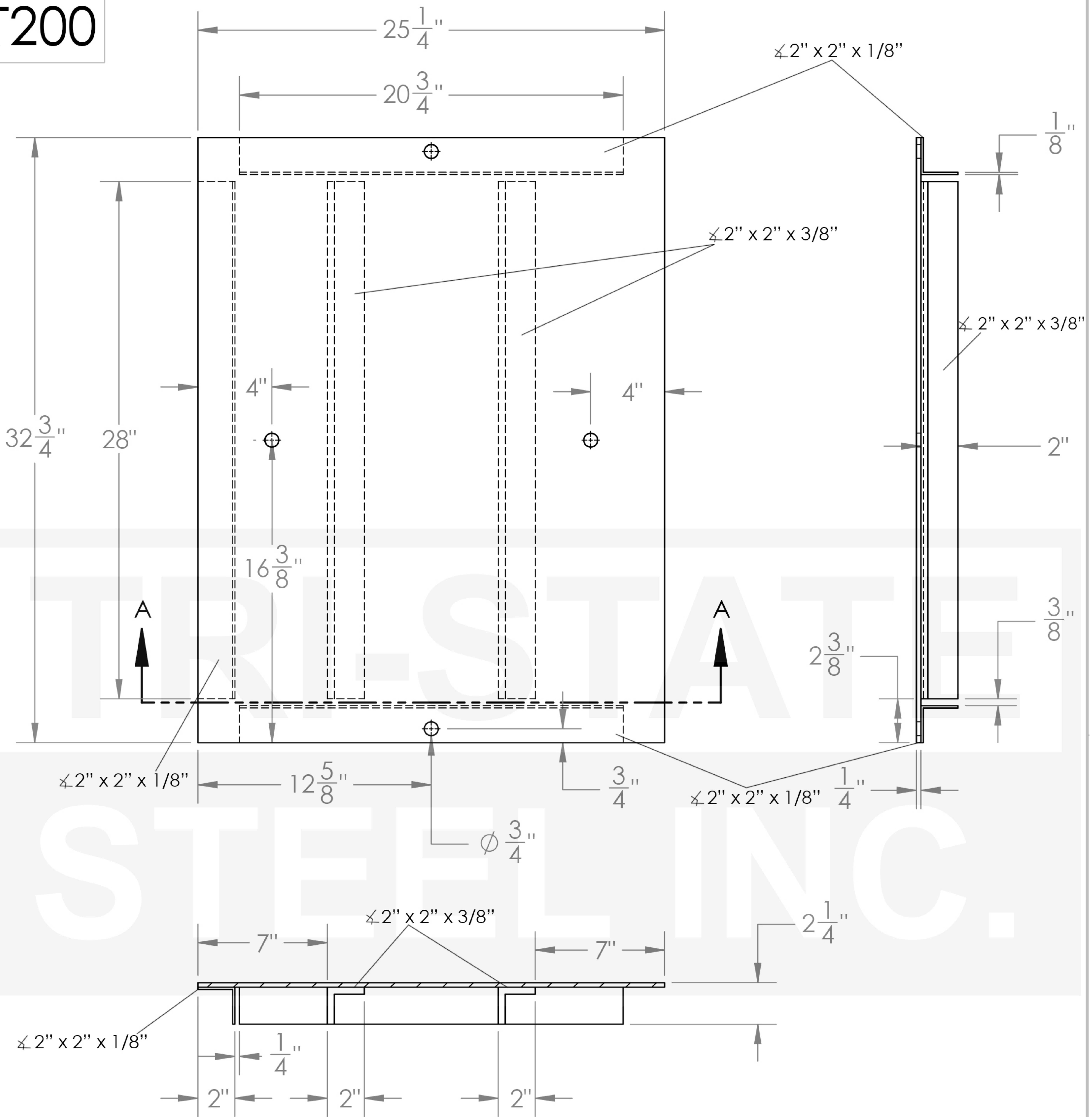
SECTION A-A
