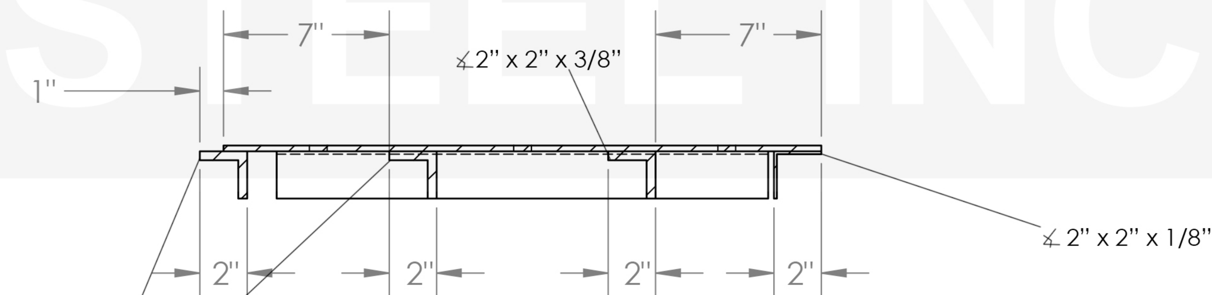
SECTION A-A
